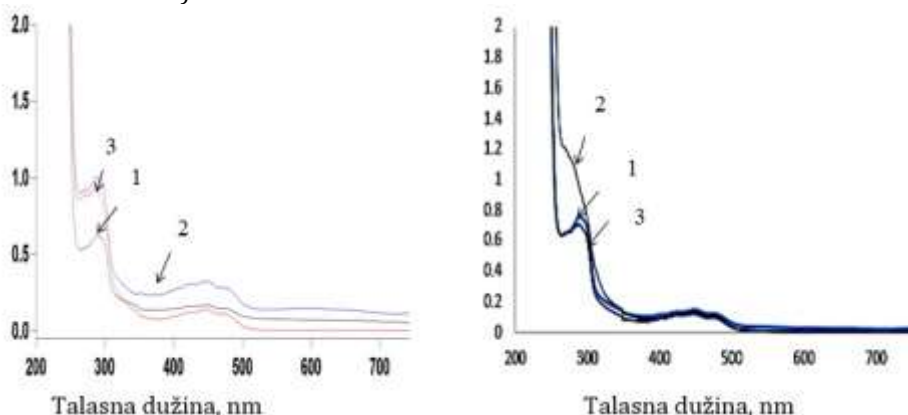
Graf. 1. Spektari različito dobijenih ulja iz lešnika pre (levo) i nakon (desno) četvoromesečnog čuvanja
